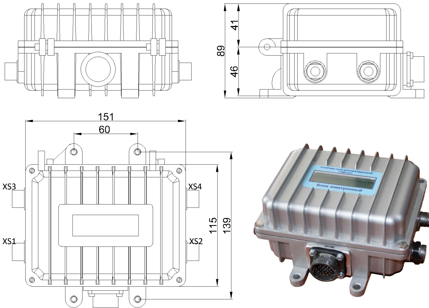
Рисунок Б.1 – Внешний вид, габаритные и установочные размеры БЭ счетчика
