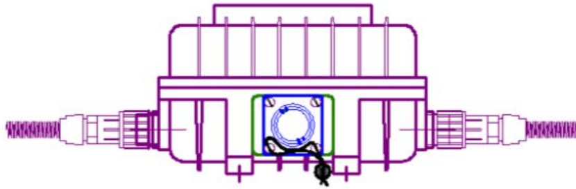
Рисунок Е.2 – Место установки пломбы при опломбировании разъема внешних подключений счетчика
