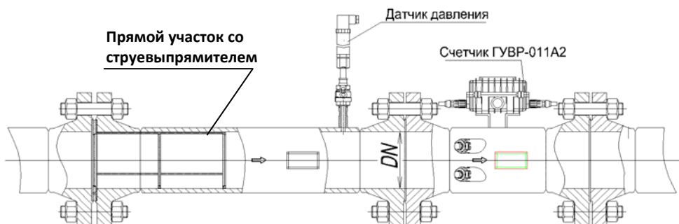
Рисунок Г.2 - Счетчик в составе: БЭ, ВС и прямой участок со струевыпрямителем
