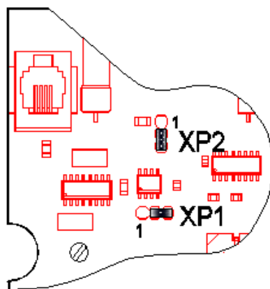
Рисунок Б.4. – Расположение штыревых соединителей на плате БПС-6.5
