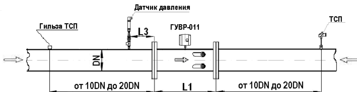
Рисунок Е.4 – Схема монтажа счетчика с байпасом, без струевыпрямителя
