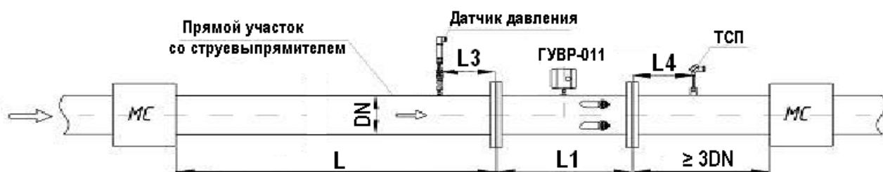
Рисунок Е.1 – Схема монтажа счетчика со струевыпрямителем
