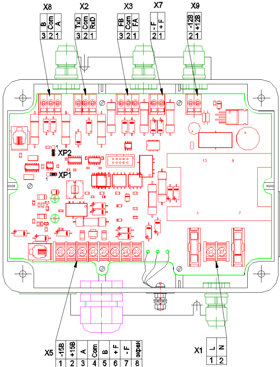
Рисунок Б.3. – Расположение клеммных колодок внешних подключений на плате БПС-6.5
