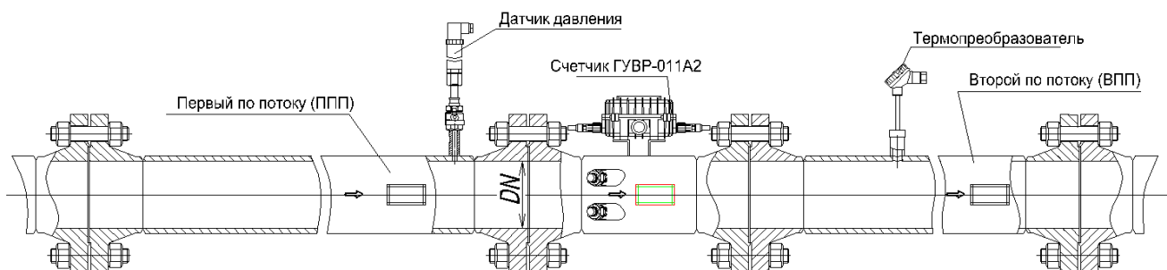
Рисунок Г.3 - Счетчик в составе: БЭ, ВС и прямые участки без струевыпрямителей до и после ВС
