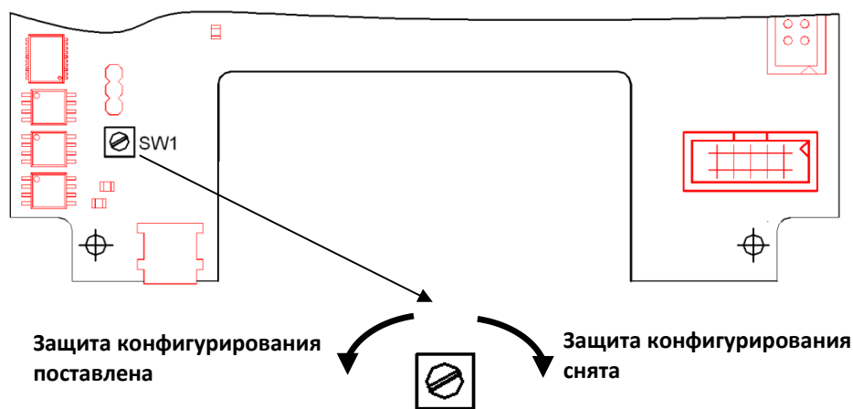
Рисунок 2 – Расположение на плате БЭ переключателя защиты конфигурации от перезаписи
