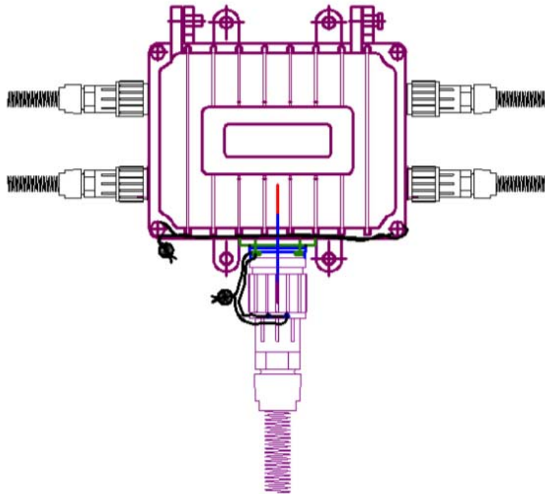
Рисунок Е.3 – Способ опломбирования корпуса БЭ и кабельной части разъема внешних подключений
